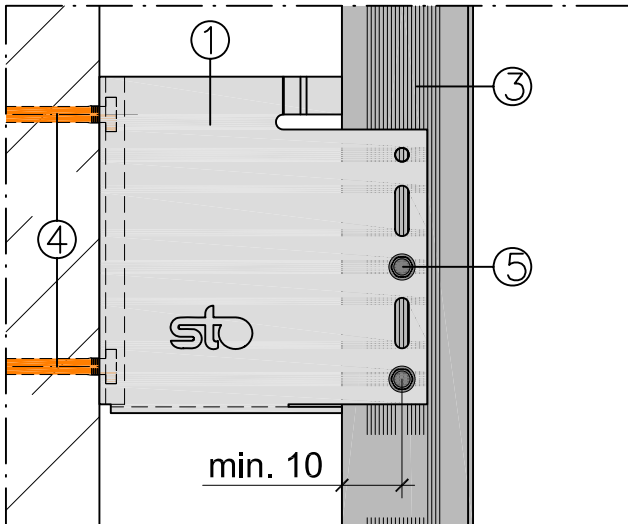
Mocowanie stałe (FP)
