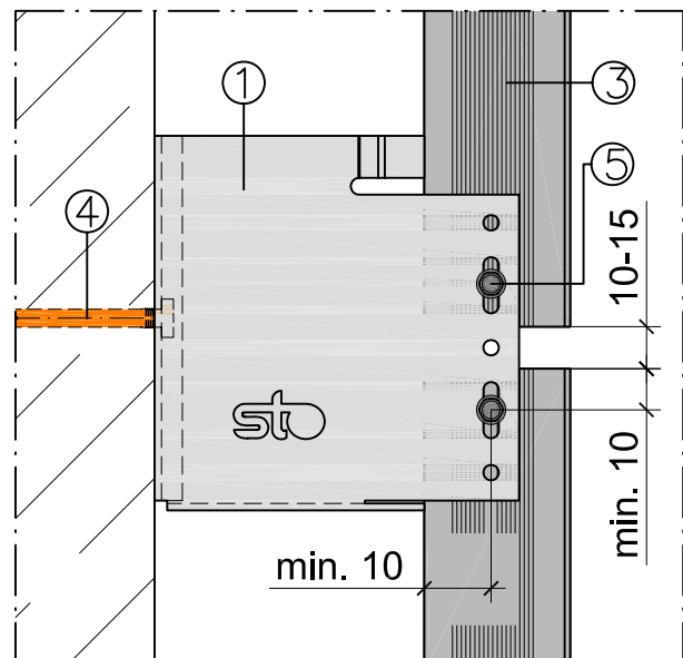
Podwójne mocowanie przesuwne (GP/GP)
