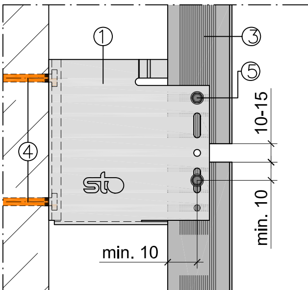
Mocowanie stało-przesuwne (FP/GP)
