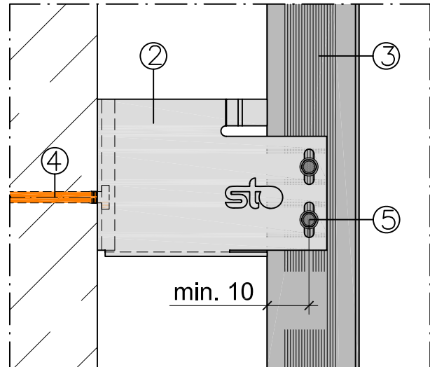
Mocowanie przesuwne (GP)
