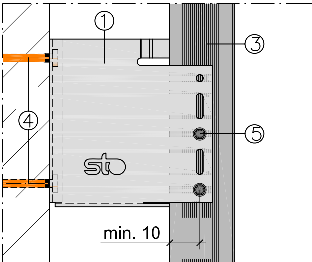
Mocowanie stałe (FP)
