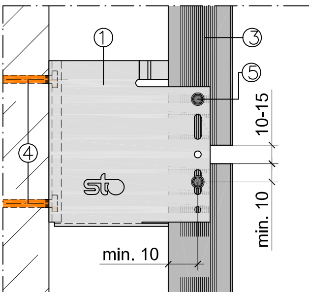
Mocowanie stało-przesuwne (FP/GP)
